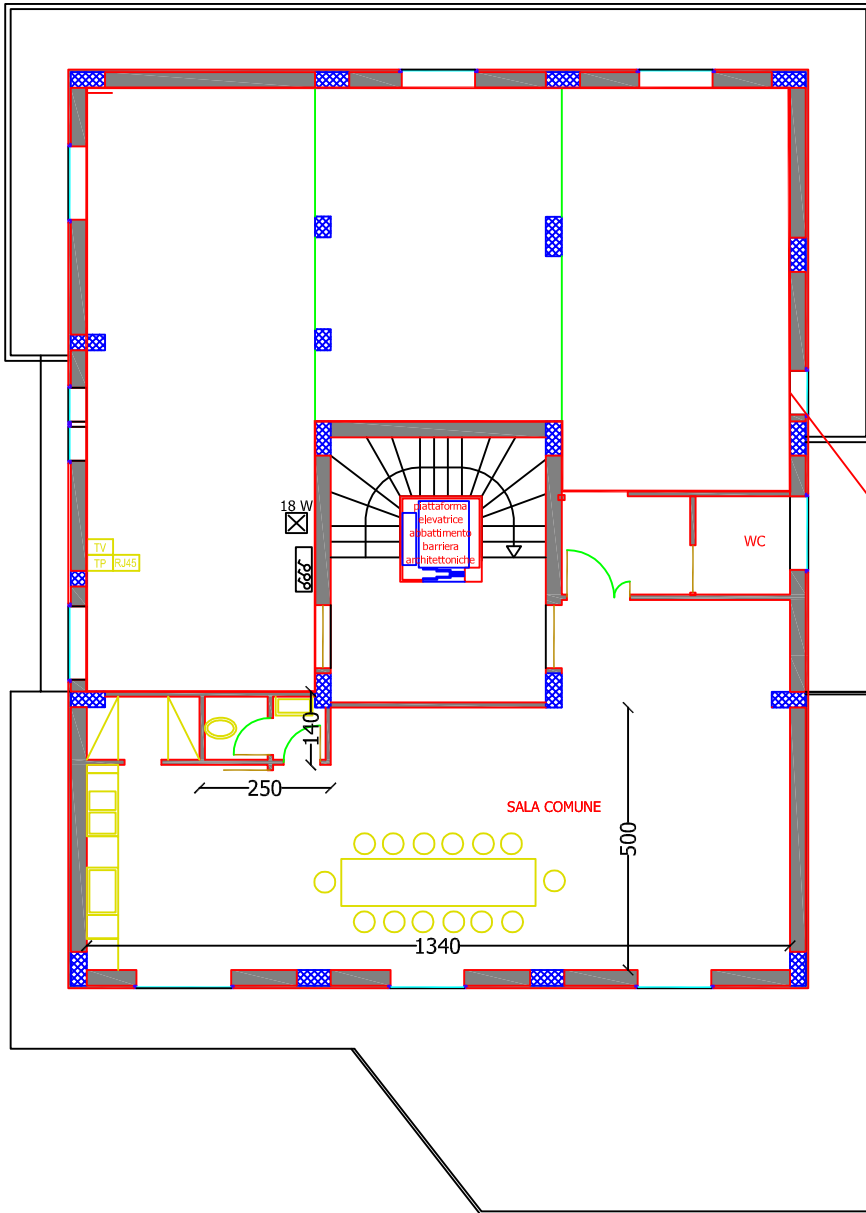
PLANIMETRIA PIANO SECONDO
