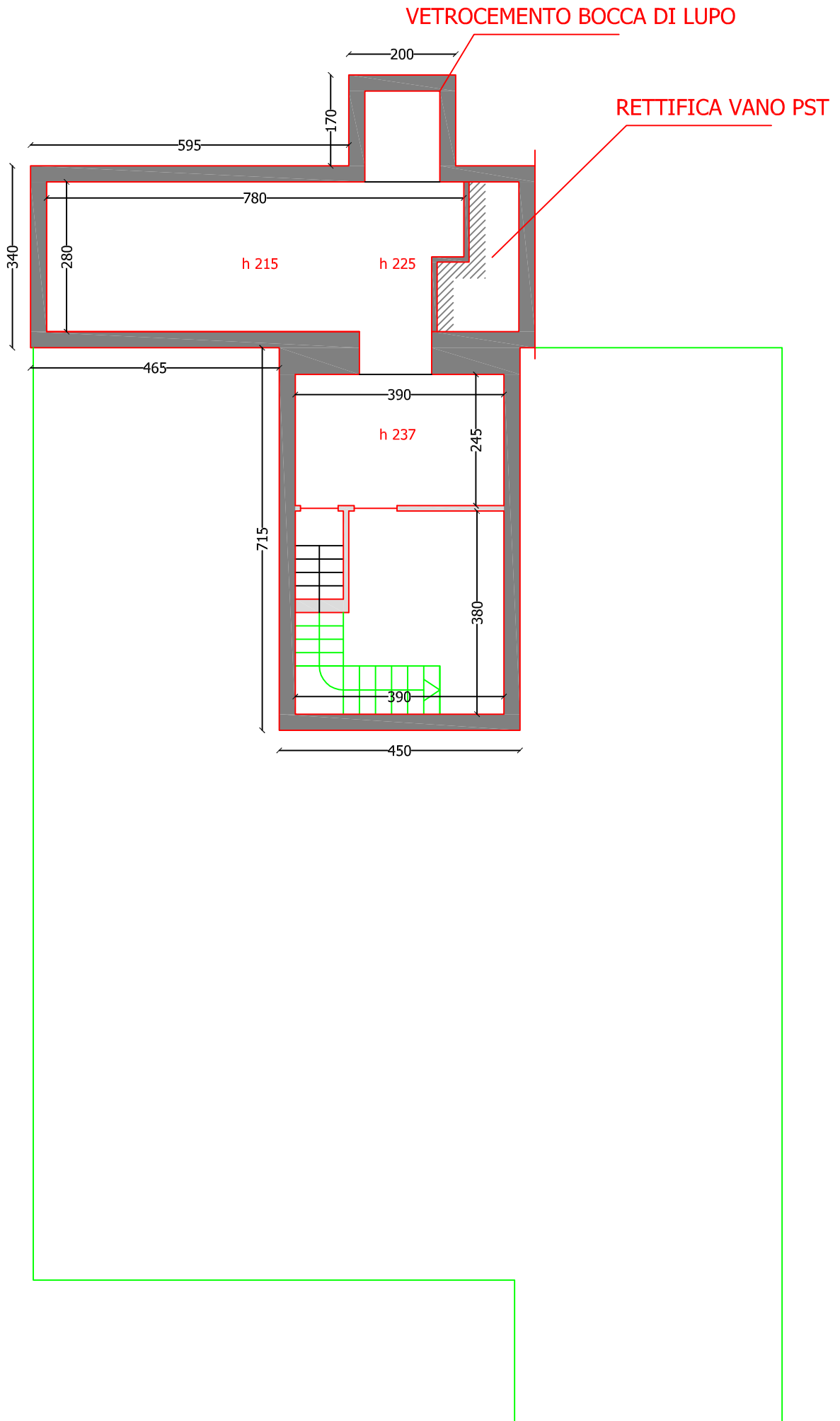
PLANIMETRIA PIANO SOTTOSTRADA
